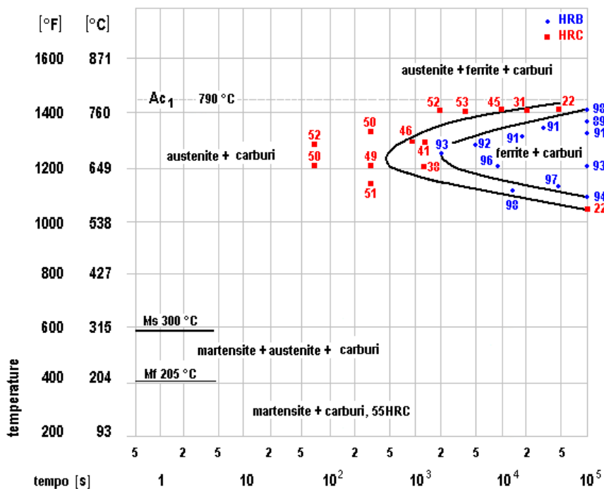
Acciaio AISI 420 diagramma T.T.T (Trasformazione – Tempo – Temperatura)
